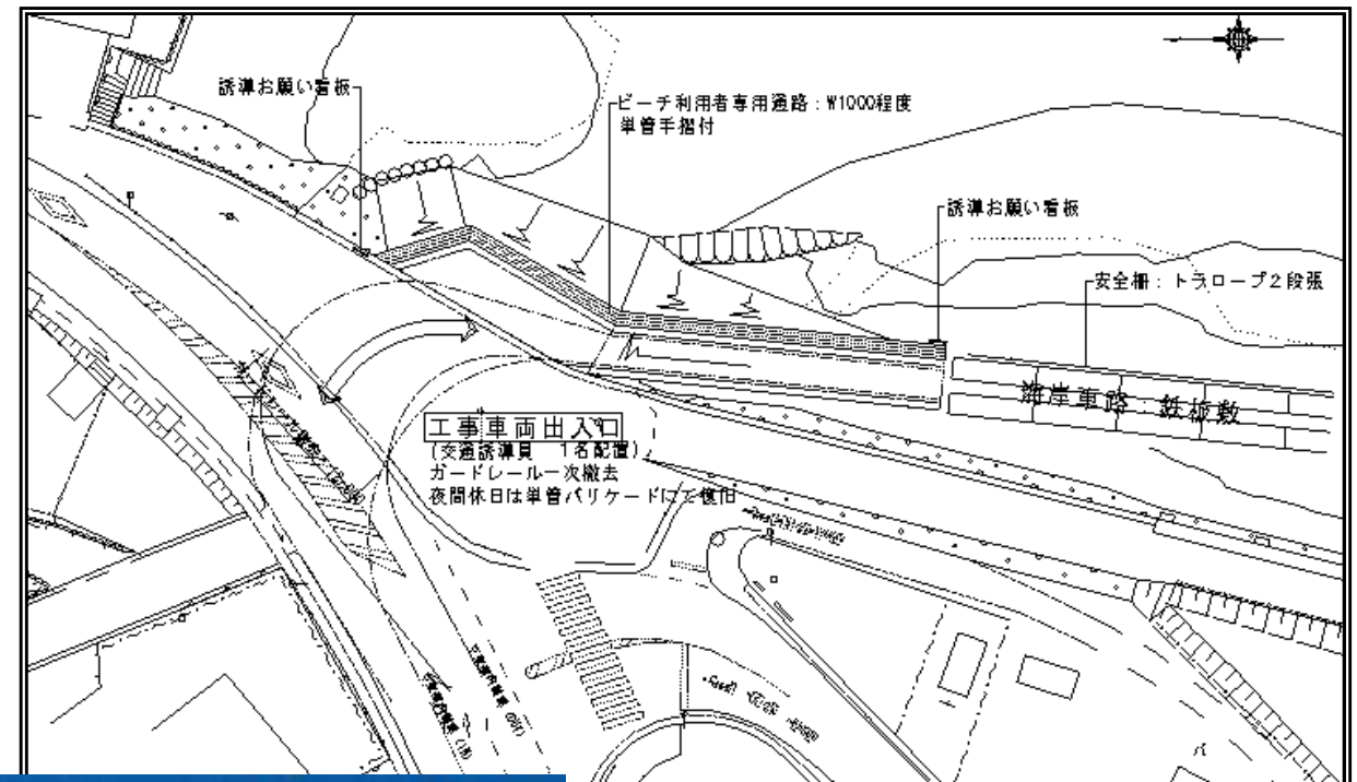
工事車両出入口計画図
